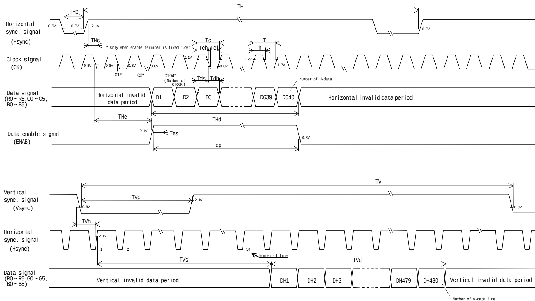
图 2 - Input signal waveforms(480 line mode)
