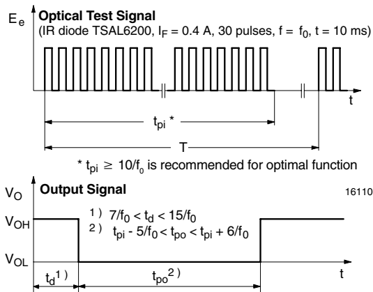
Fig. 1 - Output Function
