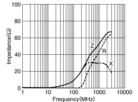
MMZ1608D800C
