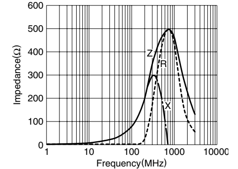
MMZ1608D800C
