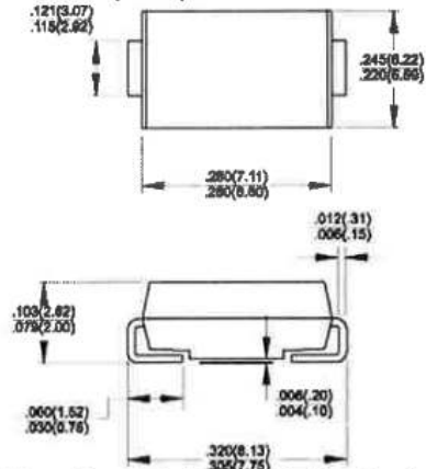
DO-214AB (SMC)
