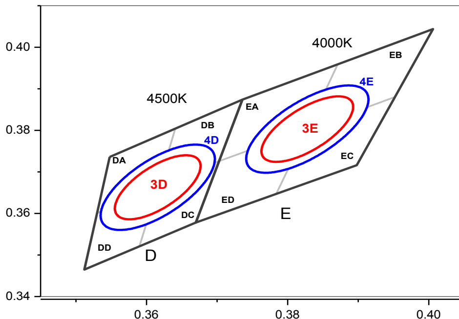
4500K 3Step
