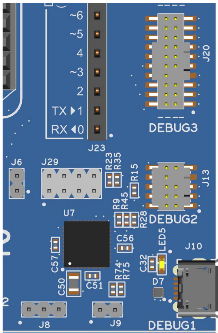
Figure 9. EK-RA4M2 Debug Interface
