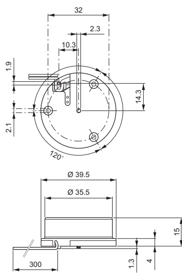
Fortimo deco mini downlight 300 827 10V
