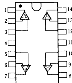
NJM2164D NJM2164M NJM2164V
