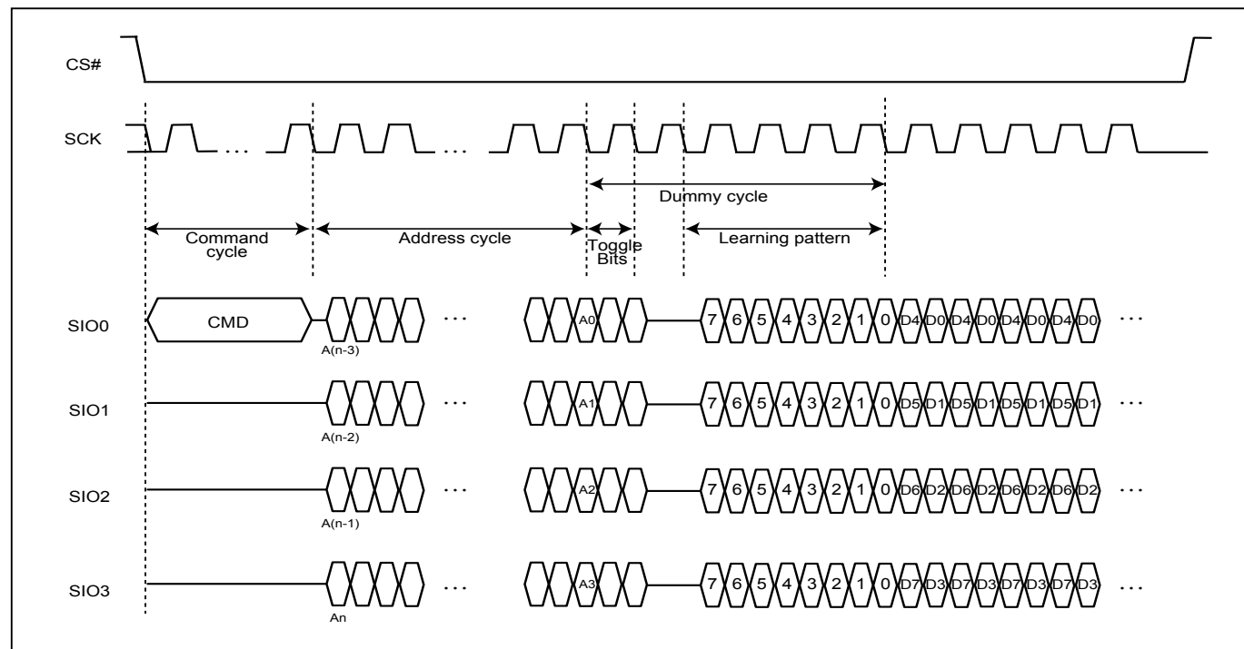
Figure 45. DTR4IO (DC=6)
