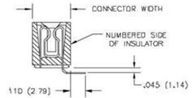
CONTACT CODE 553
