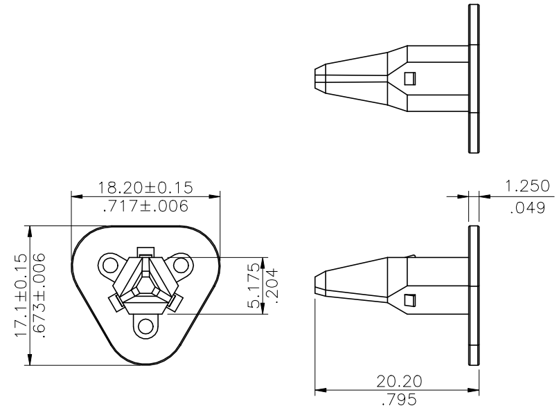
WEDGELOCK
