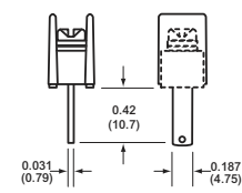
10 0.187" QC
