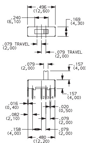
Actuator shown in pos. 3
