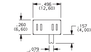
Actuator shown in pos. 3
