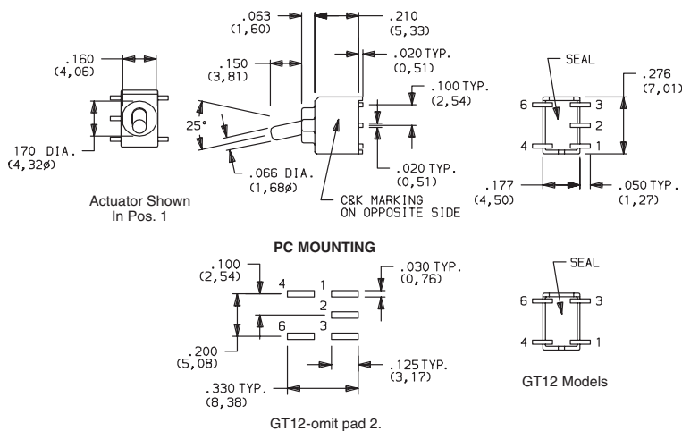
GT11MSCXE SPDT
