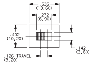
Actuator shown in pos. 3
